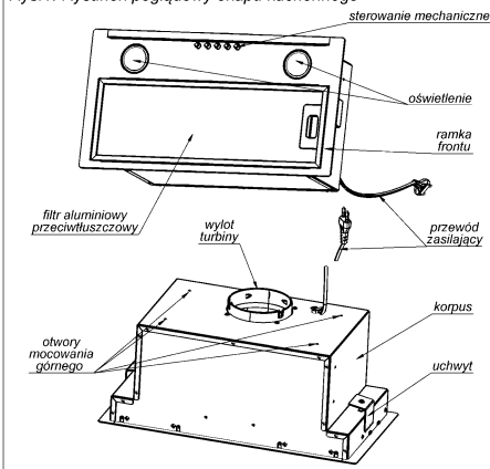
Rys. 1: Rysunek poglądowy okapu kuchennego
