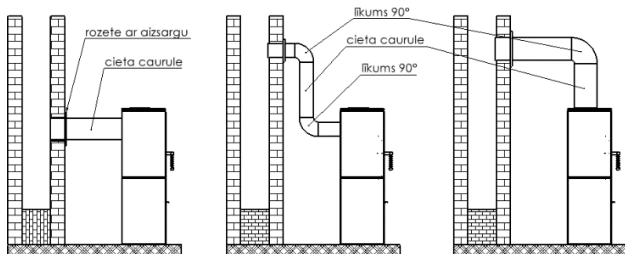
Att. 4 Kamīnkārsns pievienošanas shēma
