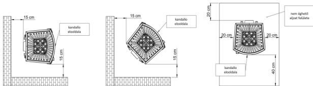
3 sz. Rajz. A kályha biztonságos távolsága a ne éghető részektől.
