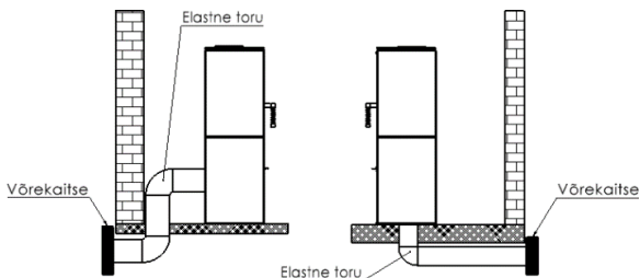
Joonis 2. Õhuvärsustuse ühenduse skeem
