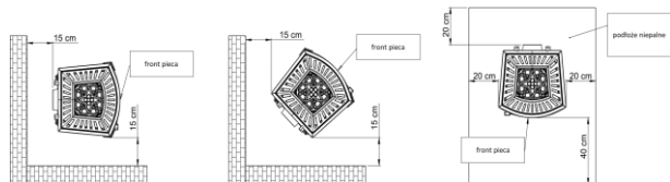
Fig.3. Trygge avstander fra ovnen til ikke-brennbare deler.
