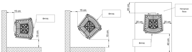
Рис. 3. Безопасное расстояние от печи до негорючих частей.
