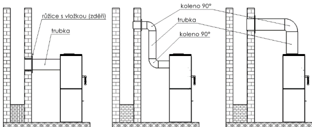
Obr.4. Schéma zapojení kamen
