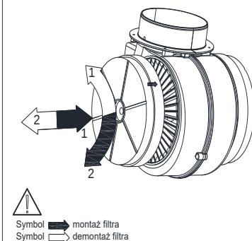
Rys. 9 Wymiana filtra węglowego.
