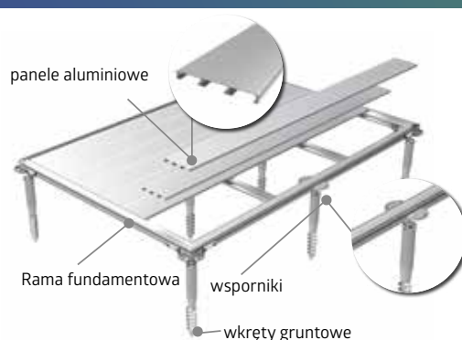
wkręty gruntowe
