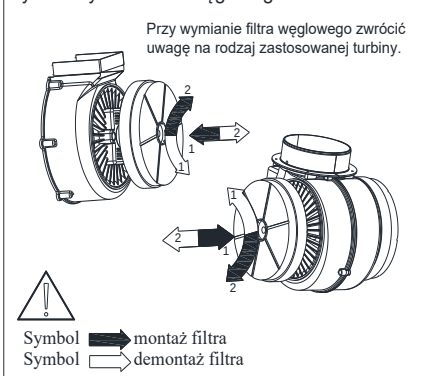
Rys.11 Wymiana filtra węglowego.
