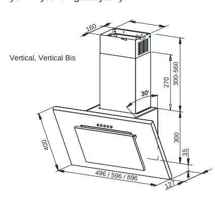
Rys. 2 Rysunek gabarytowy
