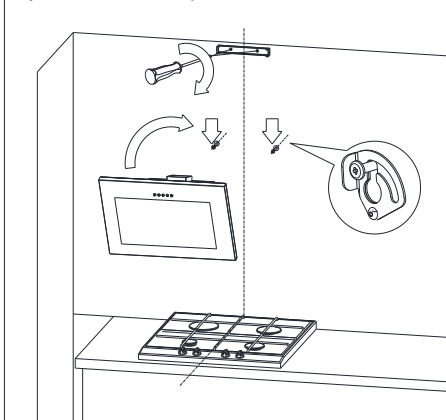
Rys. 7 Zawieszanie okapu.
