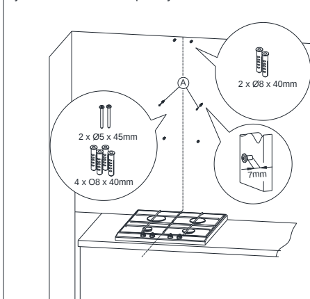
Rys. 7 Zawieszanie okapu.
