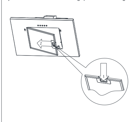
Rys. 6 Demontaż filtra aluminiowego przeciwłuszczowego.
