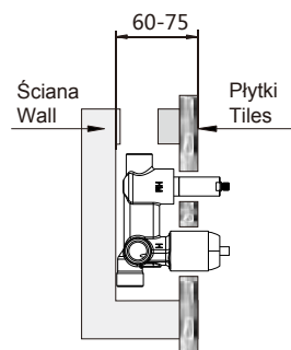
Wyjścia dla baterii 3-funkcyjnej For 3-Function outlets
