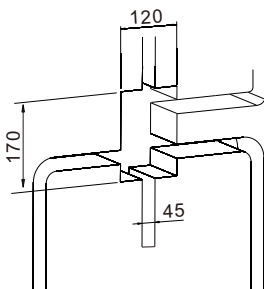
Wyjścia dla baterii 3-funkcyjnej For 3-Function outlets
