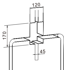
Wyjścia dla baterii 2-funkcyjnej For 2-Function outlets
